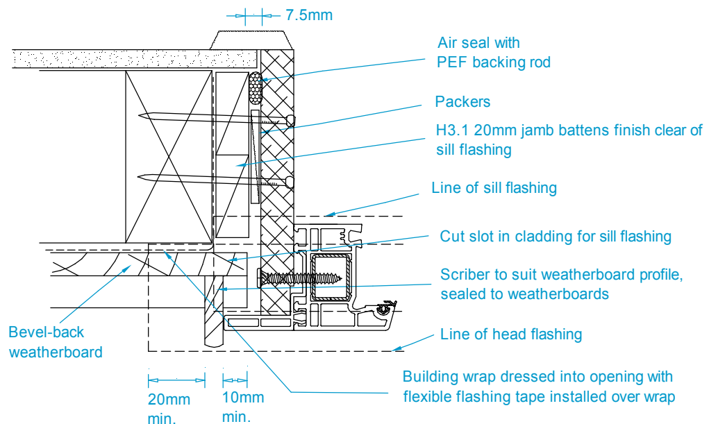
(c) JAMB
