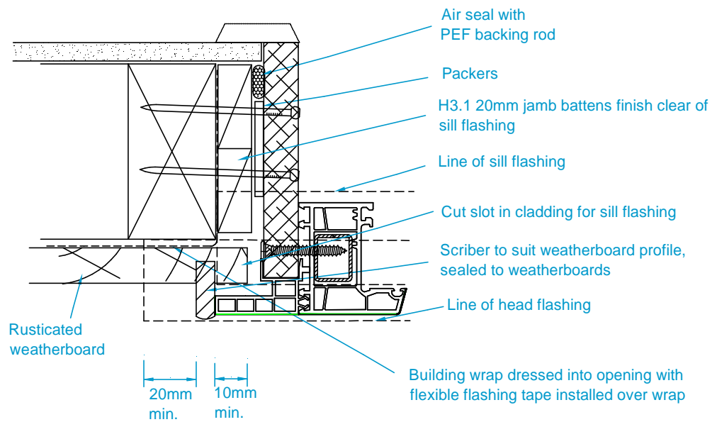
(c) JAMB
