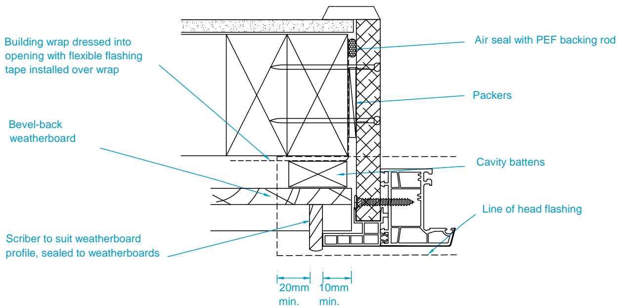
(c) JAMB
