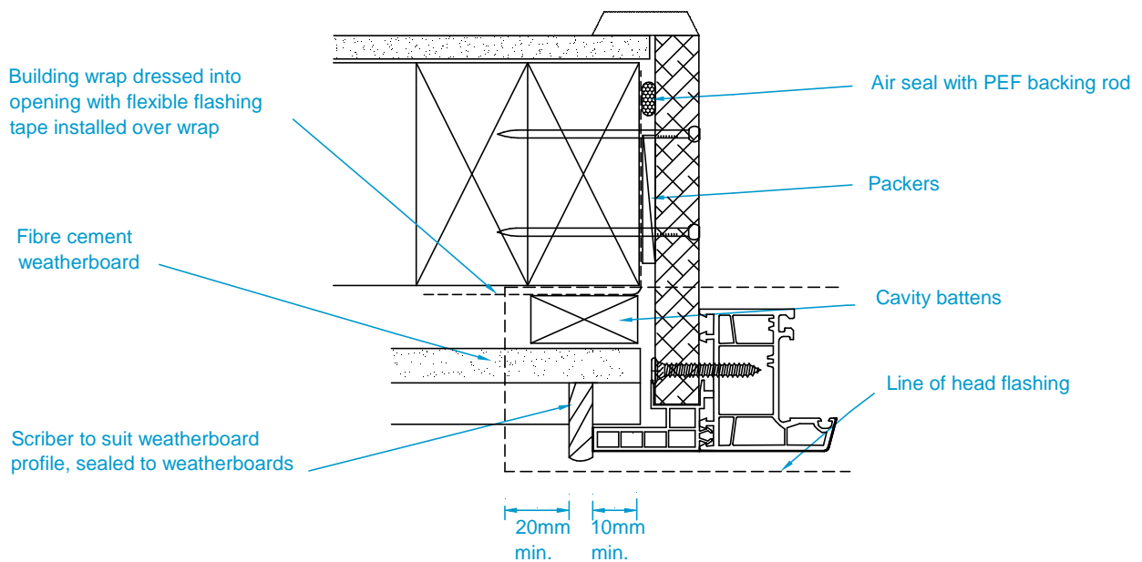
(c) JAMB
